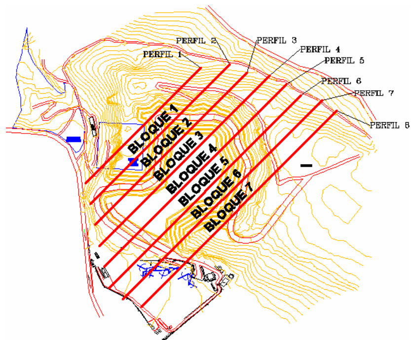
Fig. 5.2. Perfiles topográficos
