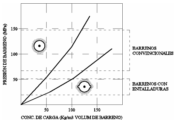
Fig. 4.10. Mejora del rendimiento de las cargas de los barrenos con entalladura (Bjarnholt y otros)
