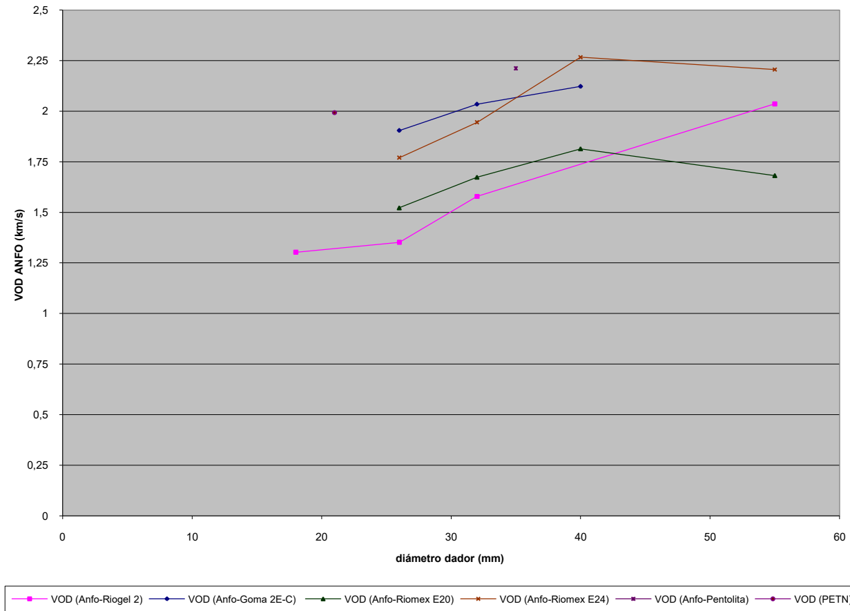
Figura 4.7 Velocidad de detonación de Nagolita iniciada con diferentes explosivos
