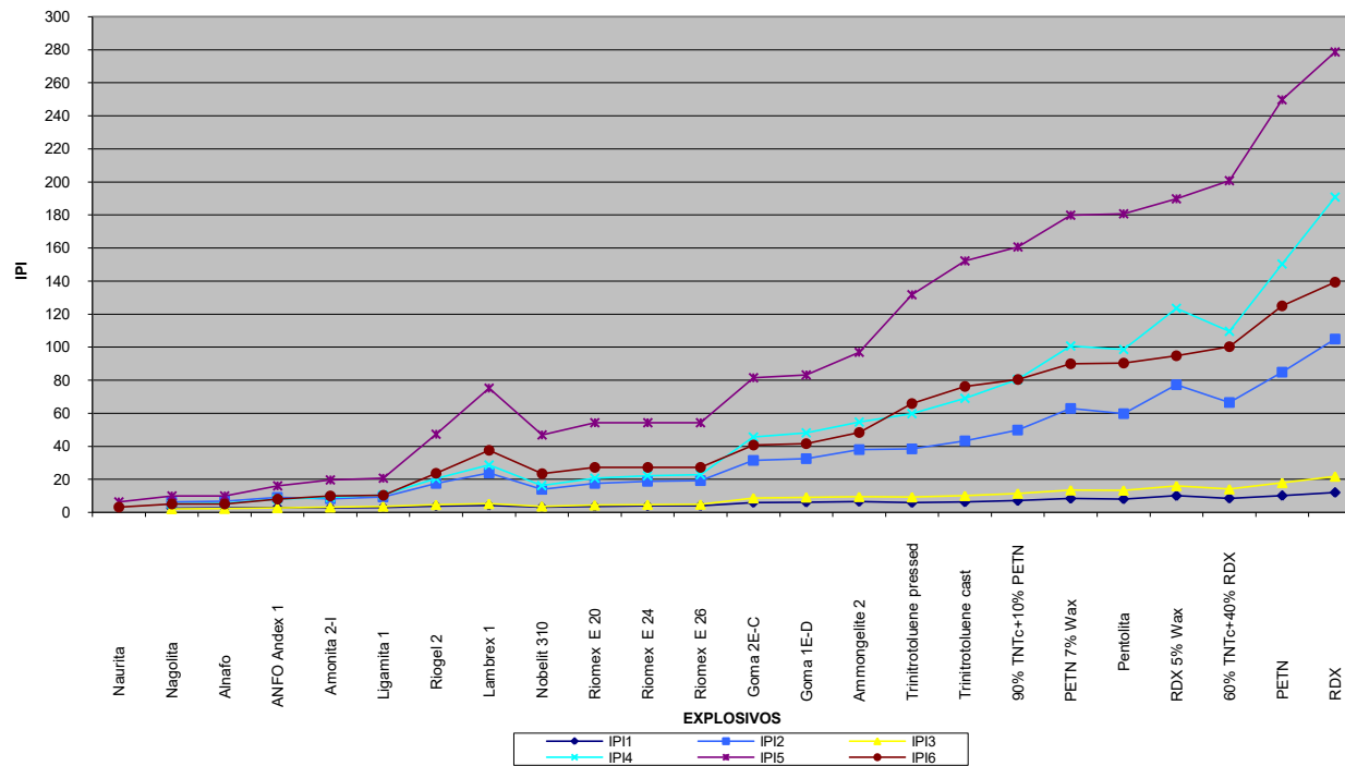
Figura 2. 7 Indices de poder iniciador
