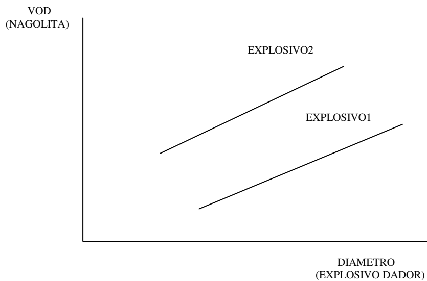
Figura 3.1. Índice de poder iniciador
