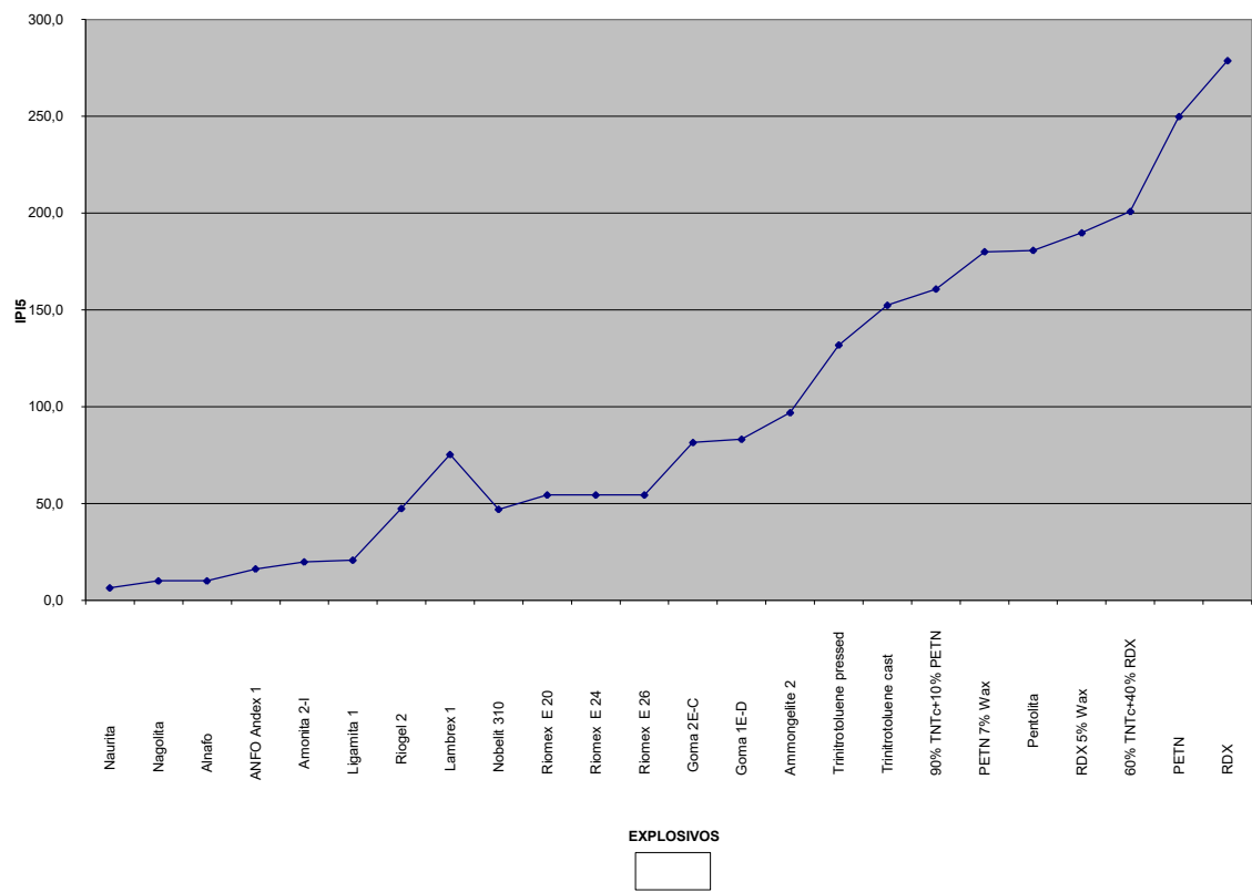
Figura 2. 5 Índice de poder iniciador 5 (IPI5)
