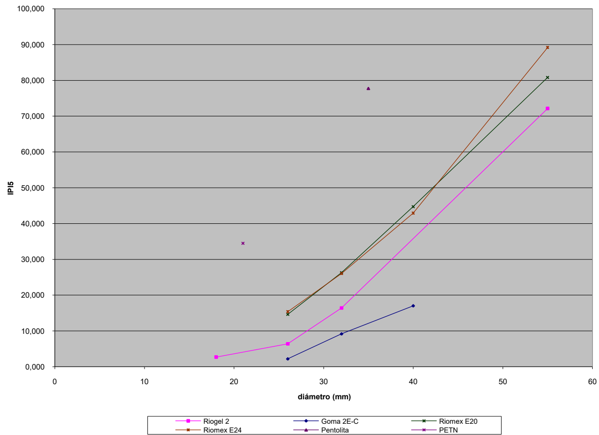
Figura 4.5 Índice de poder iniciador 5 (IPI5)
