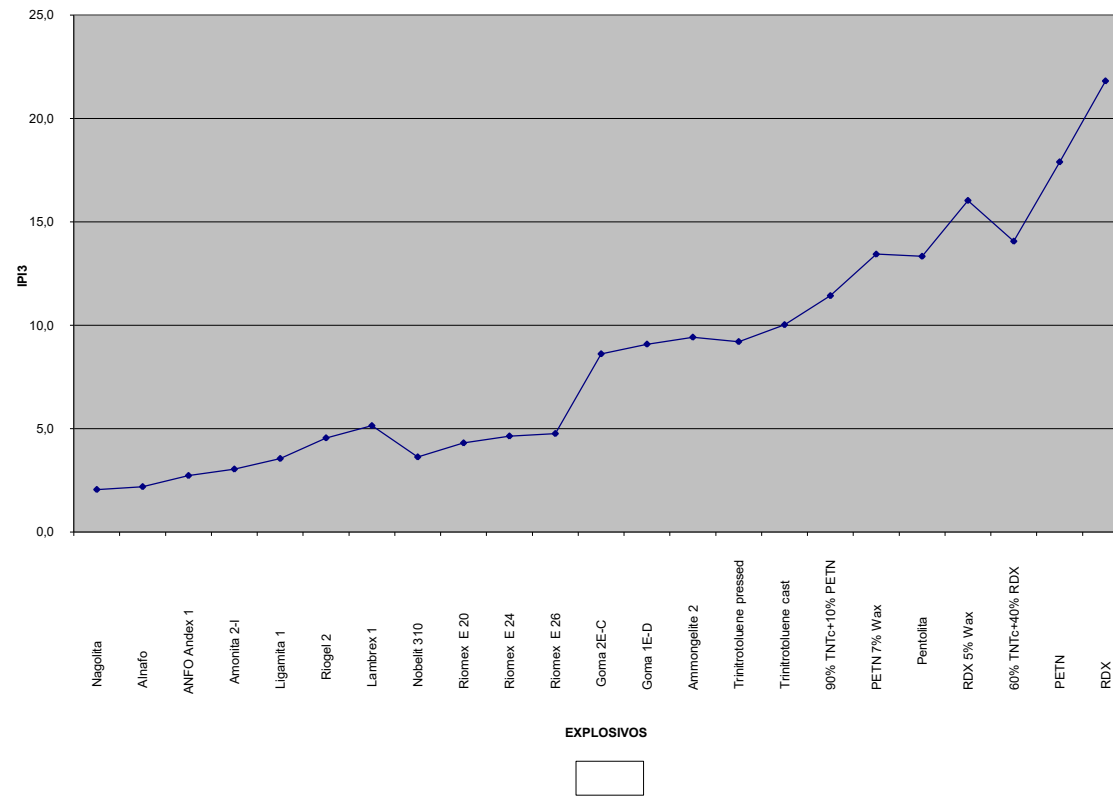
Figura 2. 3 Índice de poder iniciador 3 (IPI3)
