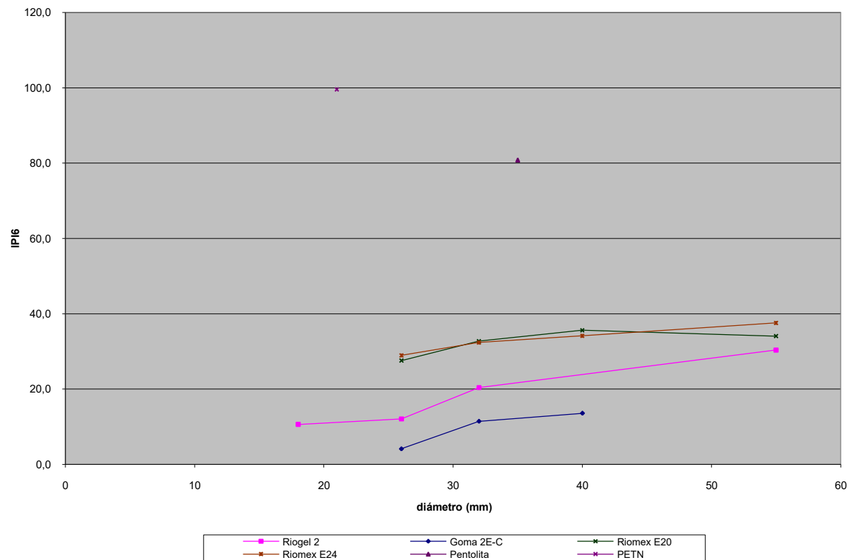
Figura 4.6 Índice de poder iniciador 6 (IPI6)
