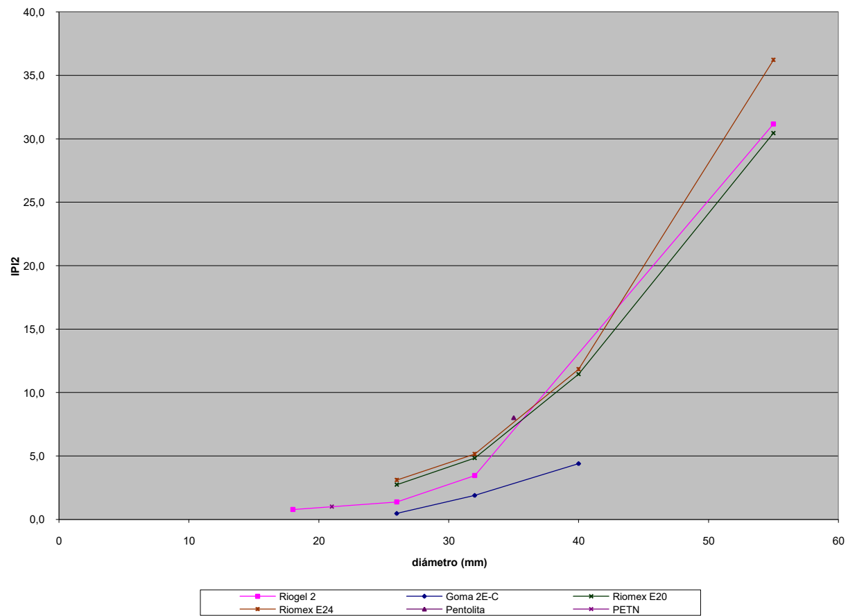
Figura 4.2 Índice de poder iniciador 2 (IPI2)
