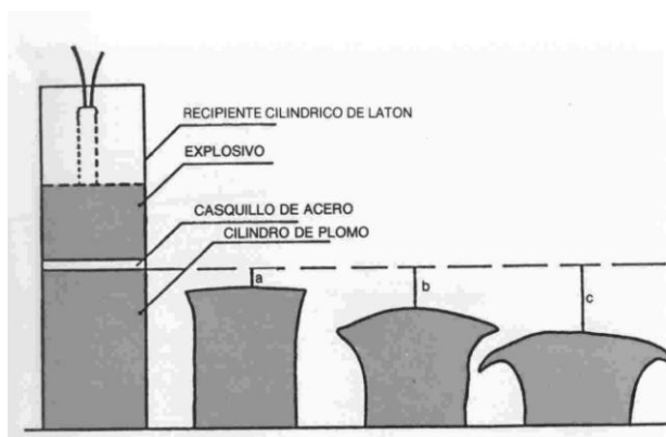
Figura 1. 14 Poder Rompedor, Método de Hess (Cortesía de UEE, S.A.)
