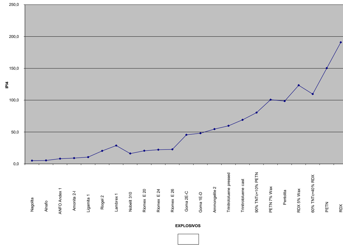
Figura 2. 4 Índice de poder iniciador 4 (IPI4)
