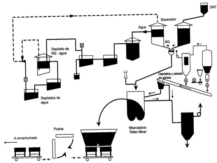
Figura 1. 2 Fabricación de explosivos gelatinosos. Teller Mixer (Curso de Tecnología de Explosivos, Sanchidrián/Muñiz)
