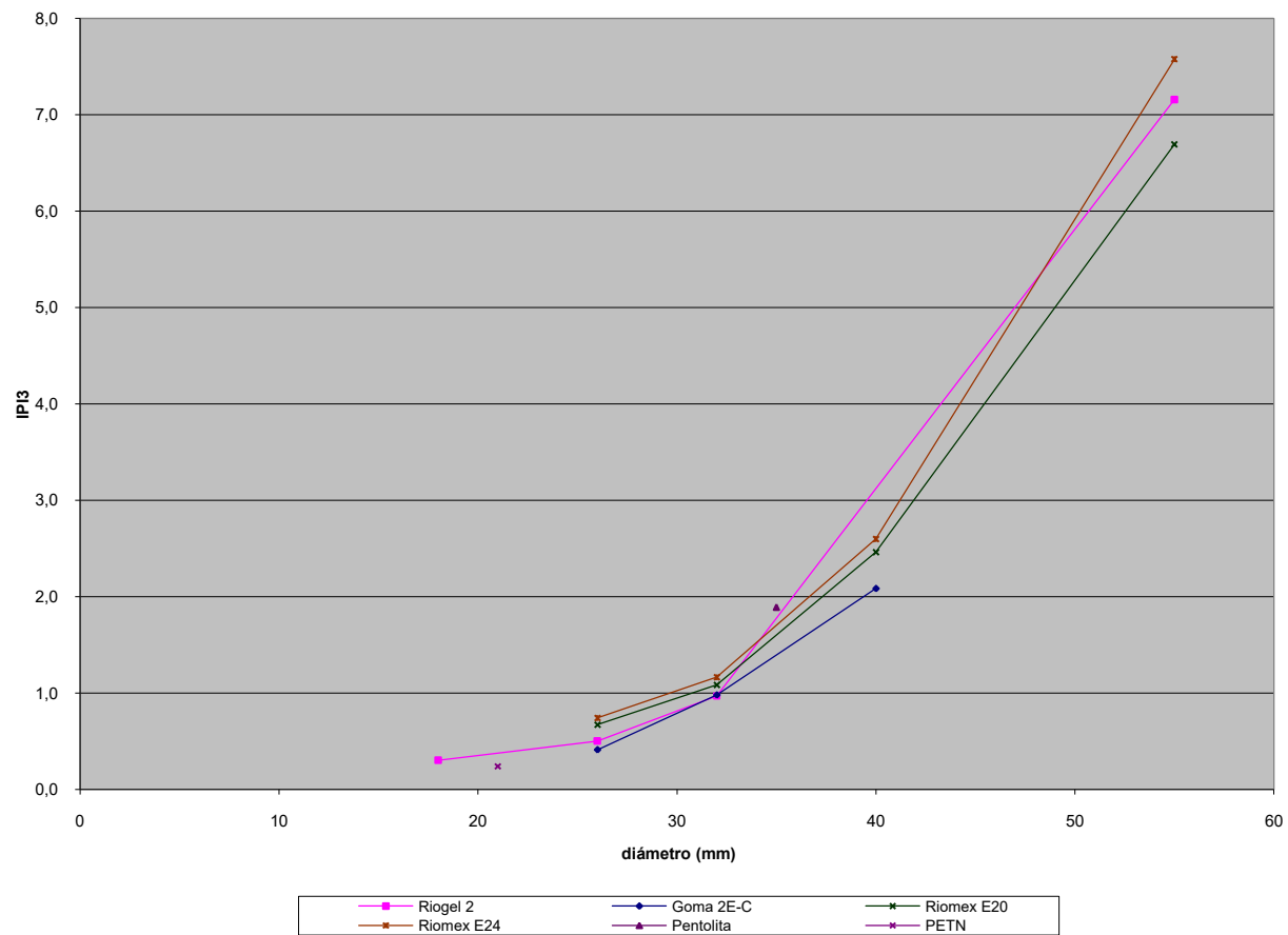
[Figura 4.3 Índice de poder iniciador 3 (IPI3)]
