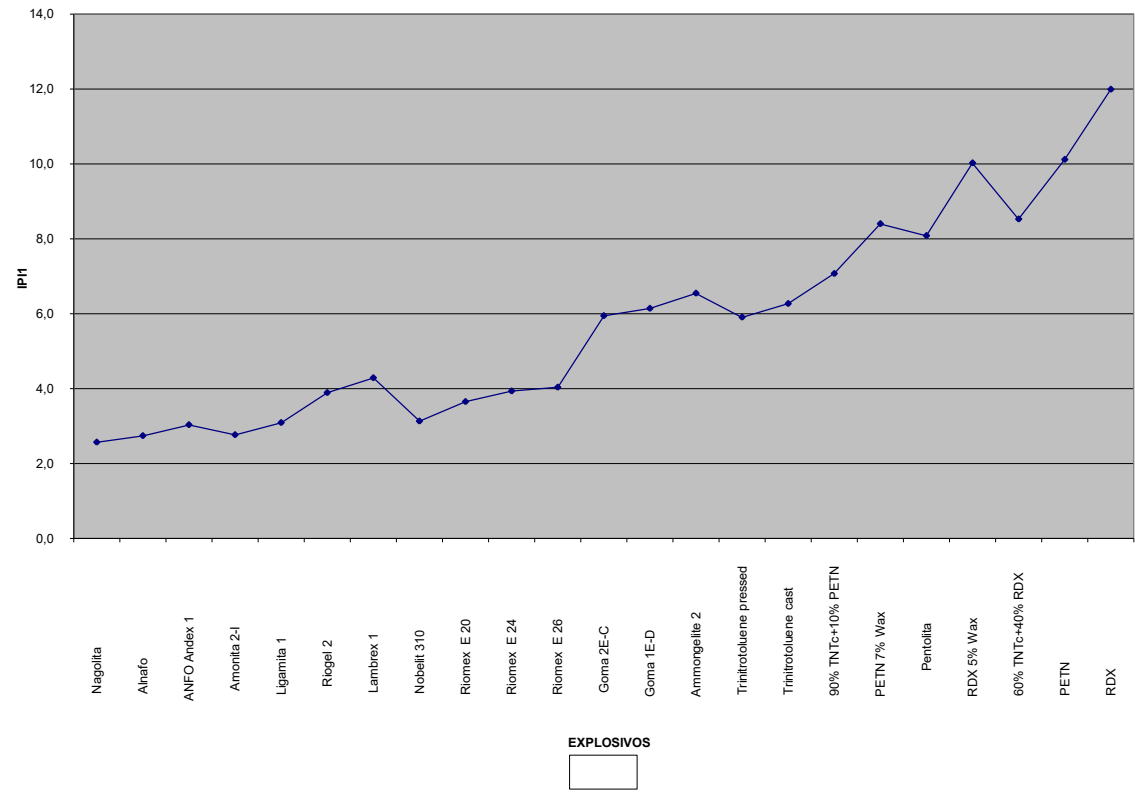
Figura 2. 1 Índice de poder iniciador 1 (IPI)
