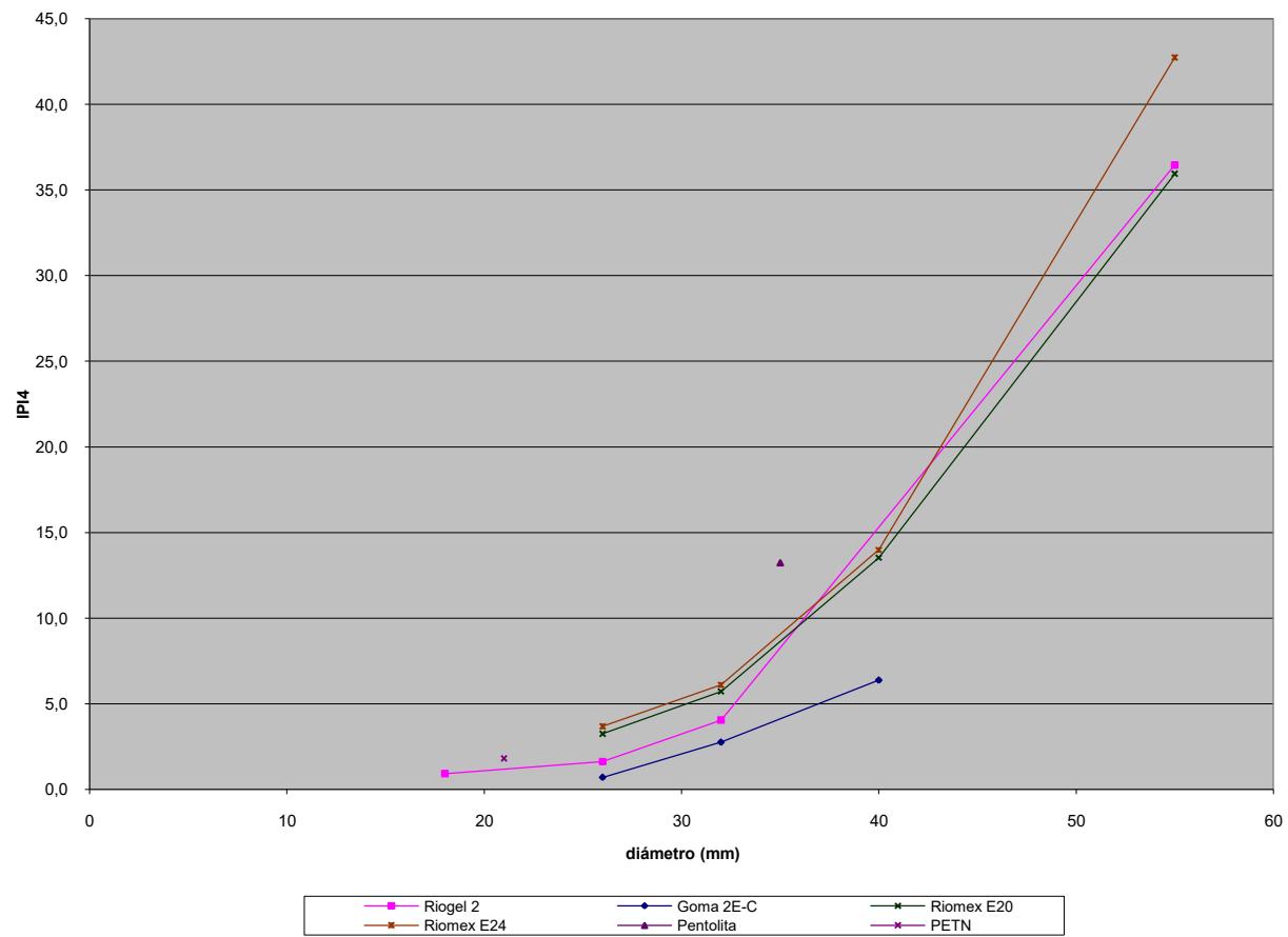
Figura 4.4 Índice de poder iniciador 4 (IPI4)
