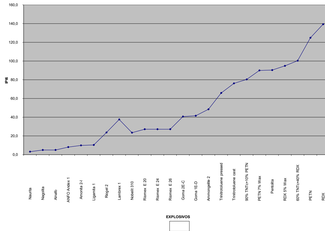
Figura 2. 6 Índice de poder iniciador 6 (IPI6)
