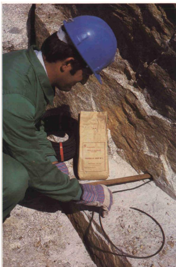
Figura 1. 12 Carga de barrenos para extracción de rocas ornamentales mediante pólvora de mina y mecha lenta (Cortesía de UEE, S.A.)
