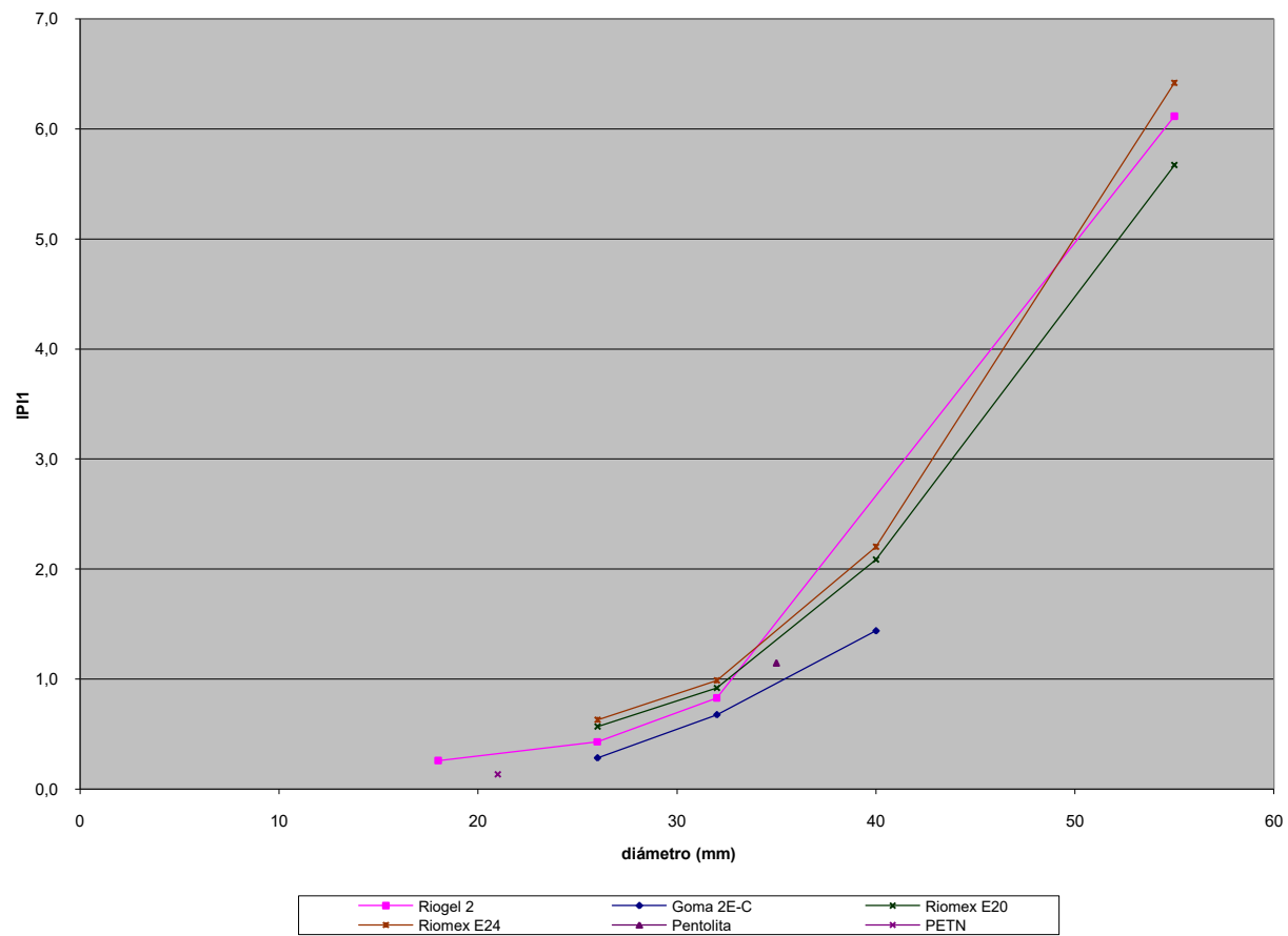
Figura 4.1 Índice de poder iniciador 1 (IPI1)
