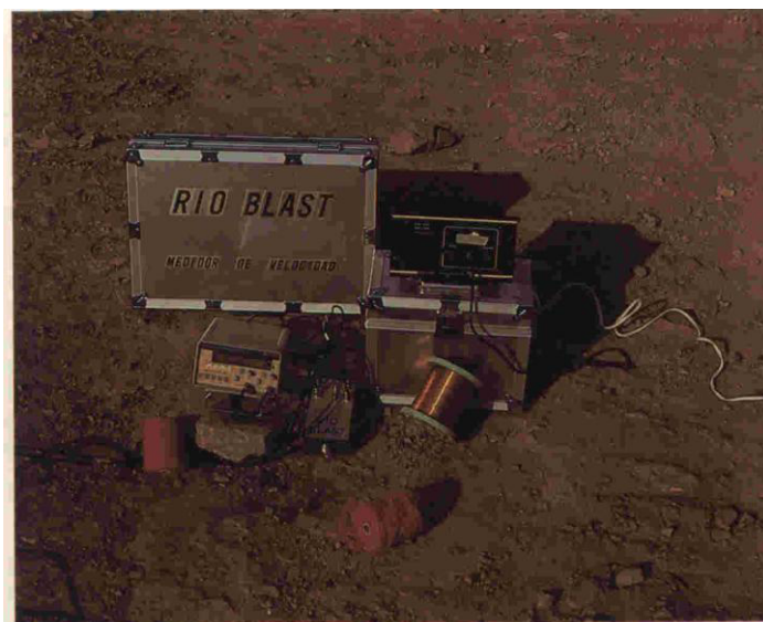
Figura 1. 15 Medidor de velocidad de detonación (Cortesía de UEE, S.A.)
