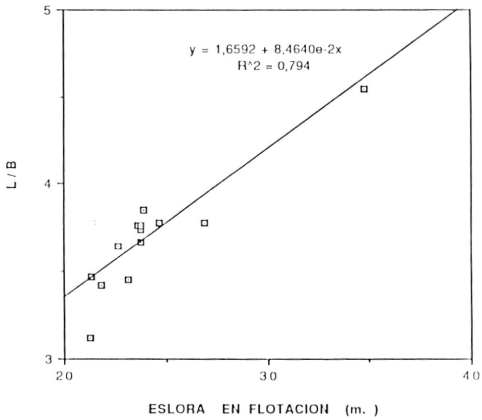
FIG.Nº34 RELACION L/B vs. ESLORA EN FLOTACION
