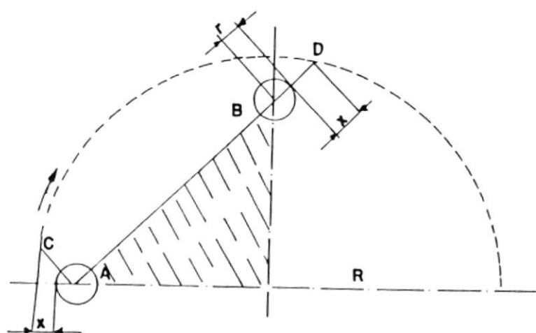
FIG. N°9 Esquema del método de Friedman
