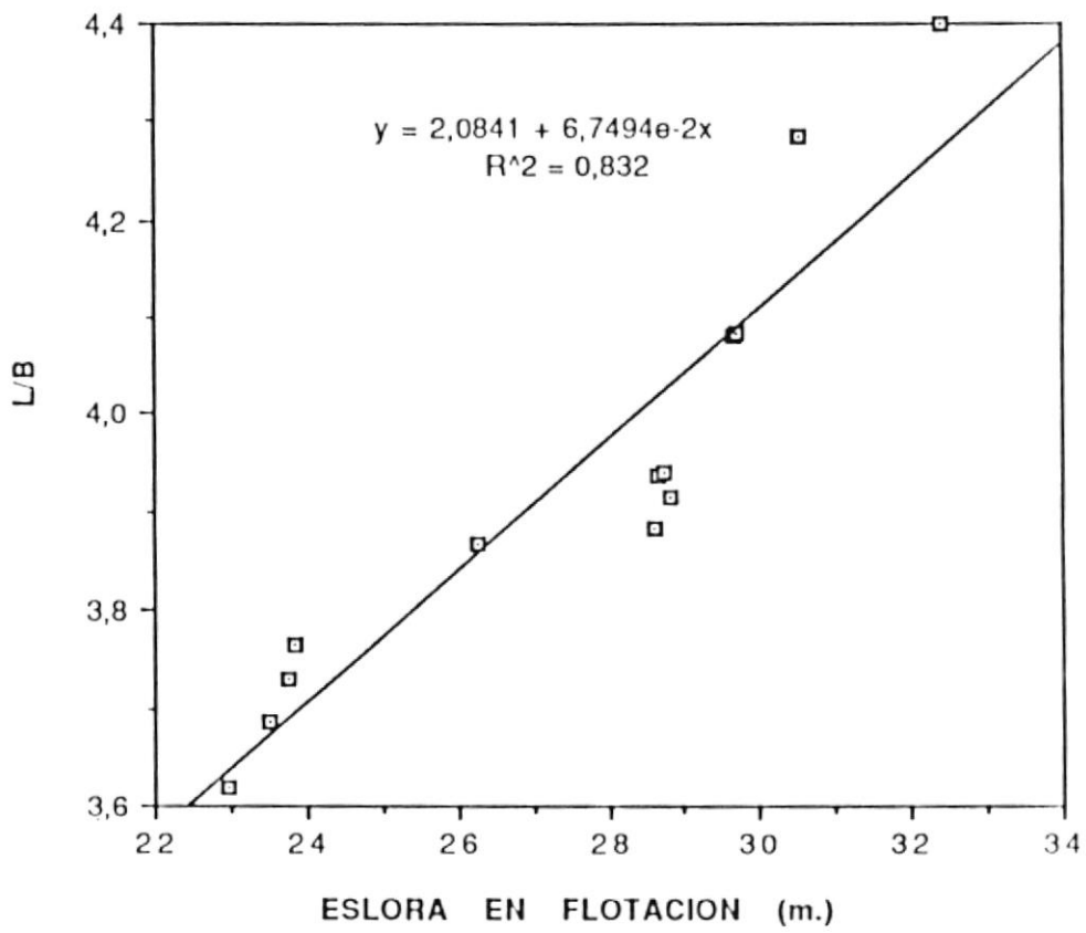
FIG. Nº39 RELACION L/B vs. ESLORA EN FLOTACION
