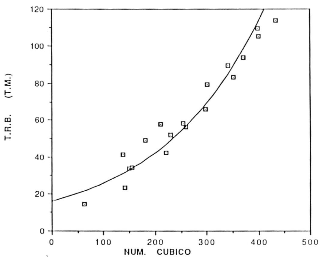
FIG. N°32 RELACION T.R.B.-NUM.CUBICO CLASE 1
