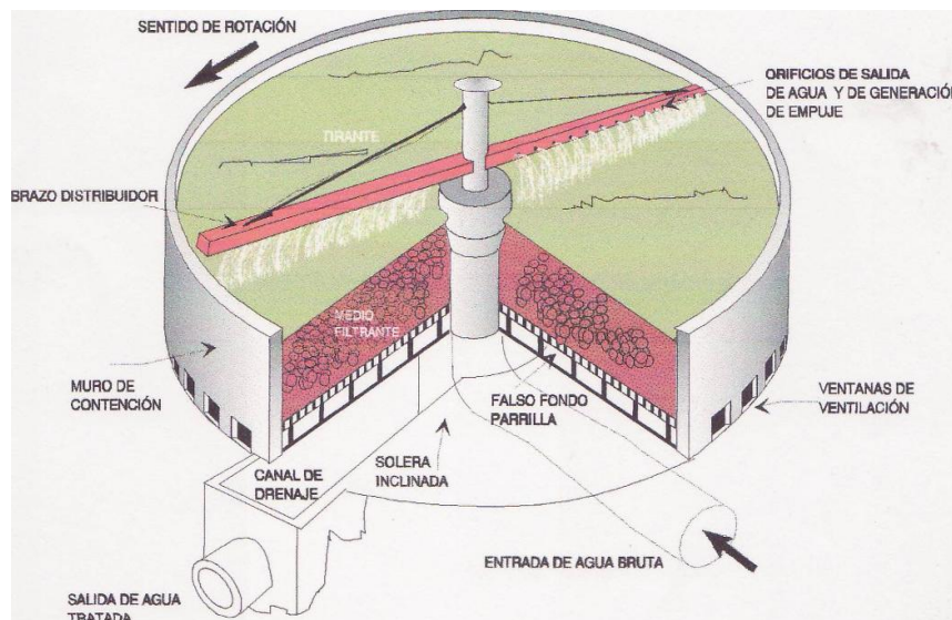
Figura 3.21. Filtro percolador o lecho bacteriano
