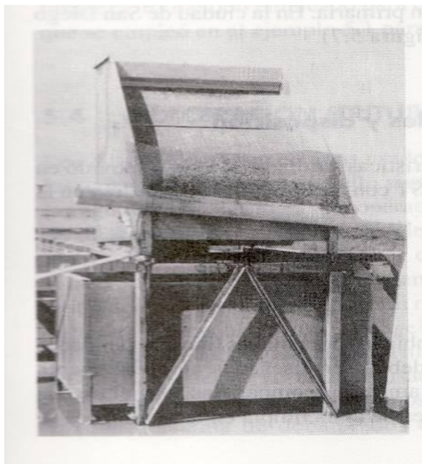
Figura 3.6. Tamiz de malla inclinada con forma de cuña.
