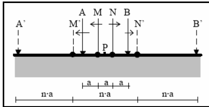
Fig. 2.12.- Método Wenner. La distancia interelectrónica pasa de a (AMNB) a n \cdot a (A'M'N'B')
