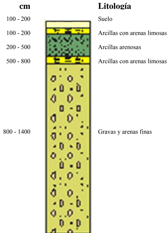
Fig. 4.1.- Columna Estratigráfica realizada en el río Olón (campo de pozos)
