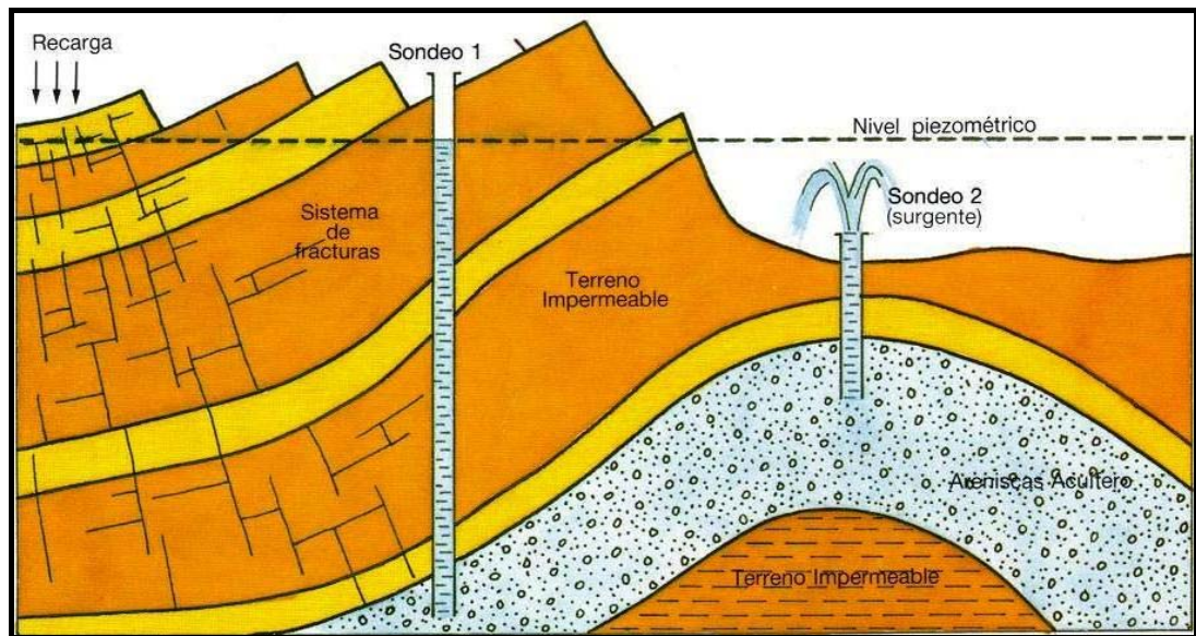
Fig. 2.5.- Acuífero Poroso-Confinado-Interior
