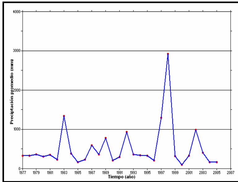
Fig. 3.1.- Precipitaciones Manglaralto
