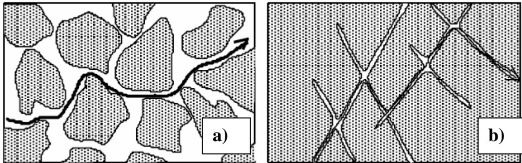
Fig. 2.2.- a) Porosidad intergranular. b) Porosidad por fracturación
