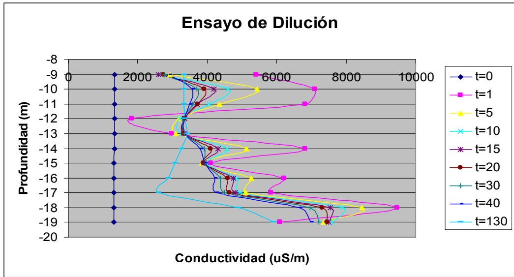
Fig 5.5.- Comportamiento del pozo.
