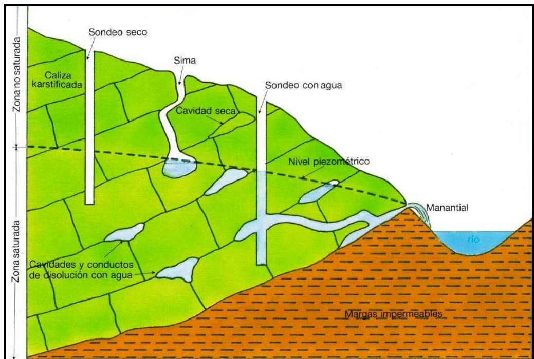
Fig. 2.4.- Acuífero Fisurado-Libre-Interior Fuente y Elaboración: IGME.
