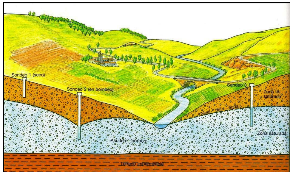
Fig. 2.3.- Acuífero Poroso-Libre-Interior Fuente y Elaboración: IGME
