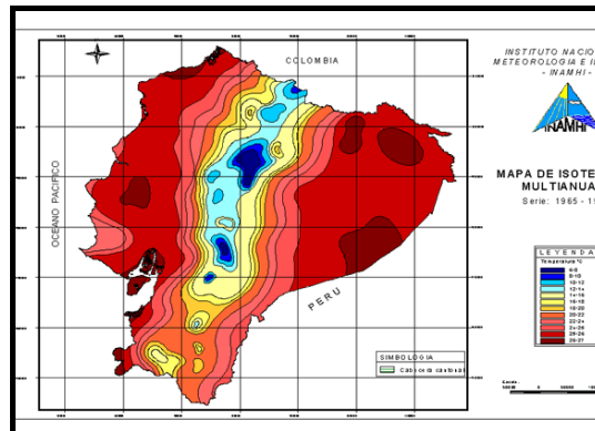
Fig. 3.3.- Mapa de isotermas Fuente y Elaboración: INAMHI.
