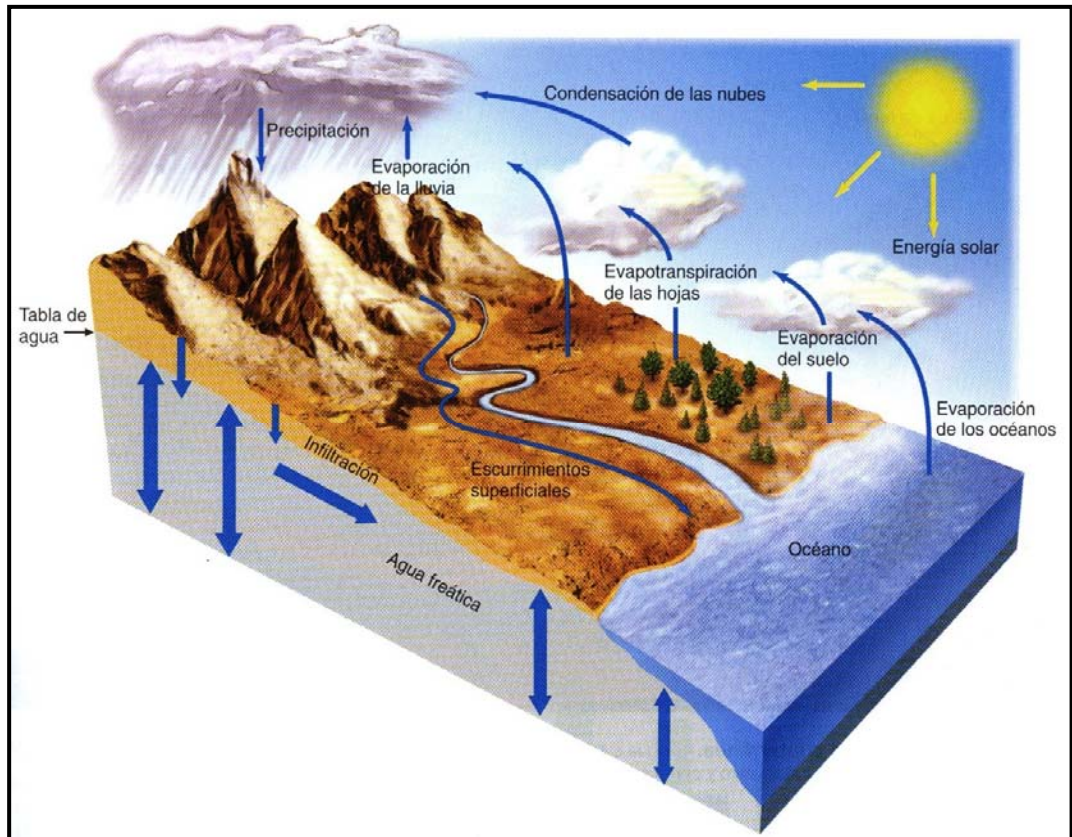
Fig. 2.1.- Ciclo hidrológico
