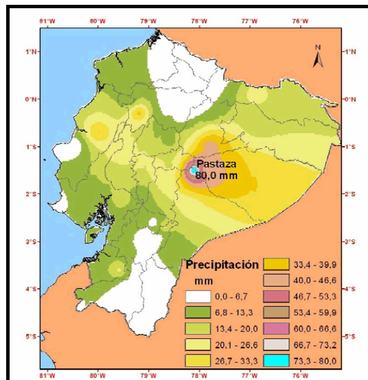
Fig. 3.2.- Mapa de precipitaciones
