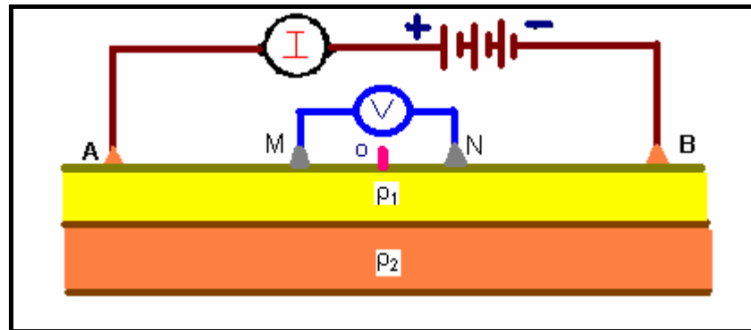
Fig. 2.9.- Método de Resistividades.
