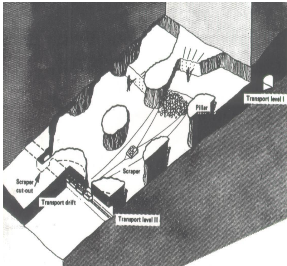
Fig. 14 Método de cámaras y pilares ( room and pillar ). En este caso los pilares siguen un espaciado regular. (Oyarzun R. Sistemas de explotación, 2005)
