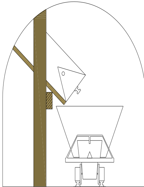
Fig. 26 Buzón de Acumulación de mineral ( Crespo J. 2007 )
