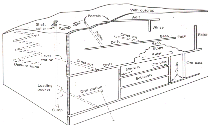
Fig. 9 Distintos elementos constitutivos de una mina subterránea. (Oyarzun R. Sistemas de explotación, 2005)
