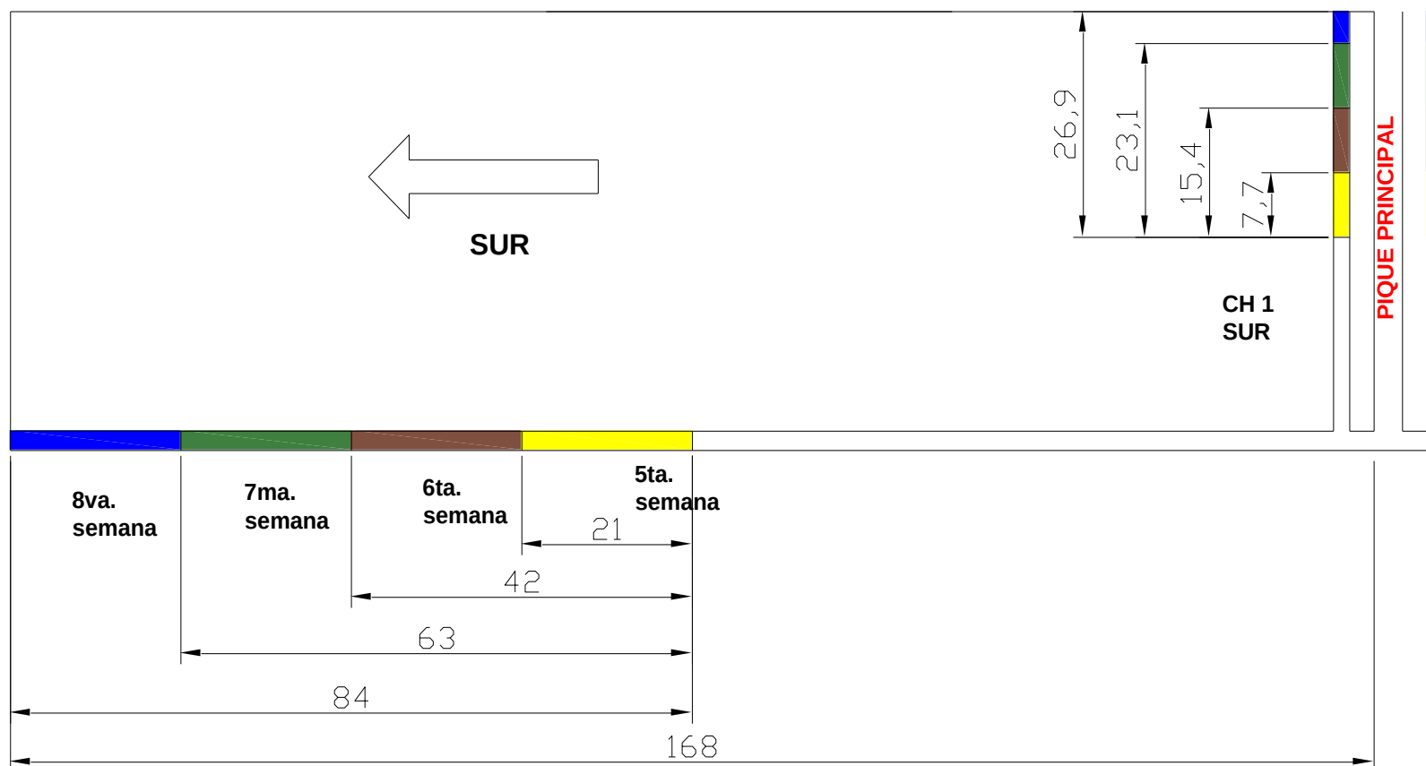
Fig. 36 Avance lineal de 5ta Semana a 8va Semana Sur ( Crespo J. 2007 )
