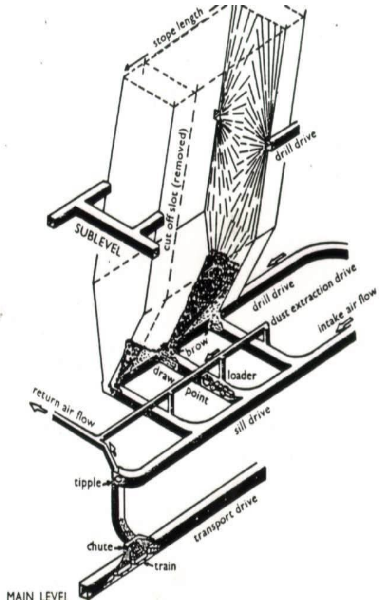
Fig. 13 Longhole stoping. Note el diagrama de disparo en abanico desde dos galerías. (Oyarzun R. Sistemas de explotación, 2005)
