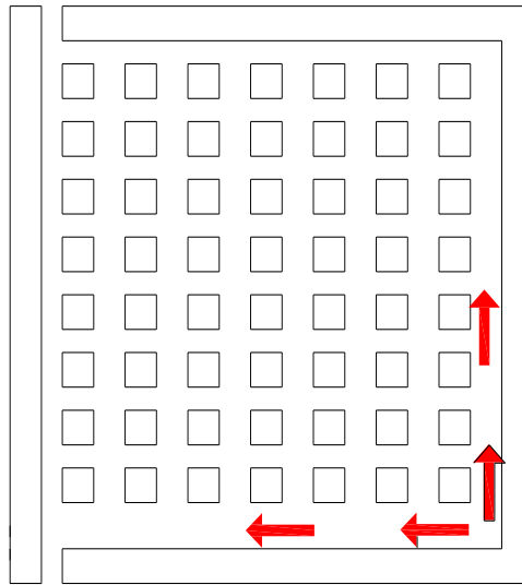
Fig. 23 Extracción de pilares en retirada ( Crespo J. 2007)
