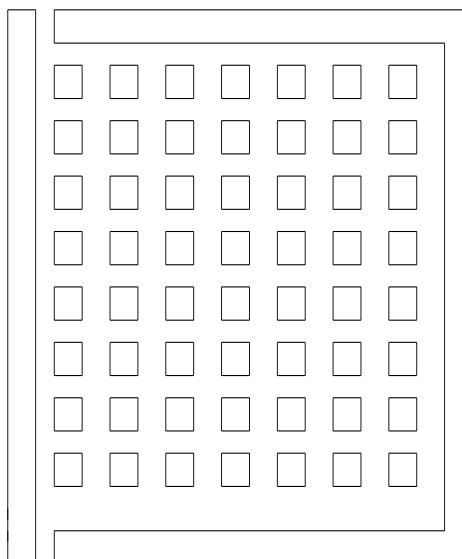
Fig. 21 Geometría del bloque utilizando cámaras y pilares ( Crespo J. 2007)
