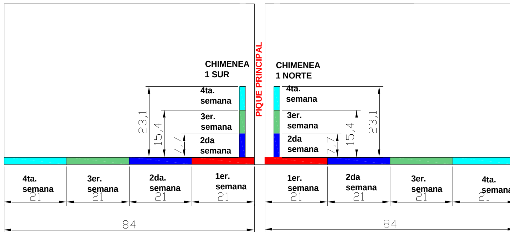
Fig. 35 Avance lineal de 1era Semana a 4ta Semana (Crespo J. 2007)
