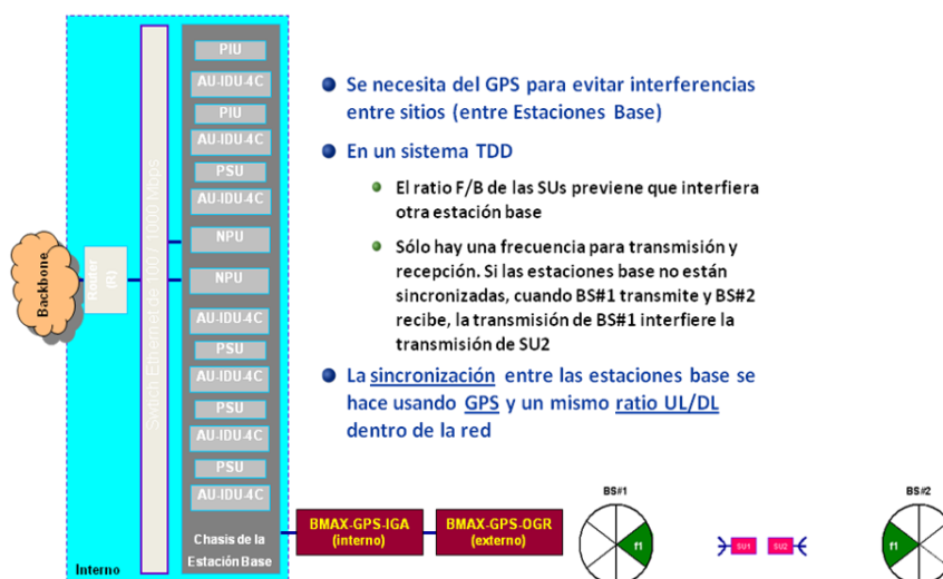
Fig. 4.29.- Sistema de Sincronización mediante GPS.
