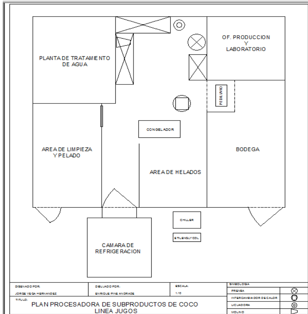
Plano 2. Diseño planta propuesta (autocad 2008).
