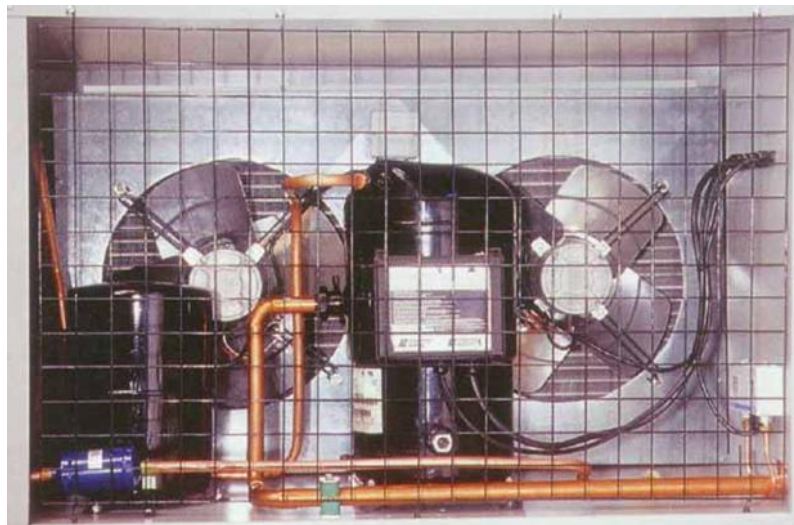
Figura 3.9 Condensador.
