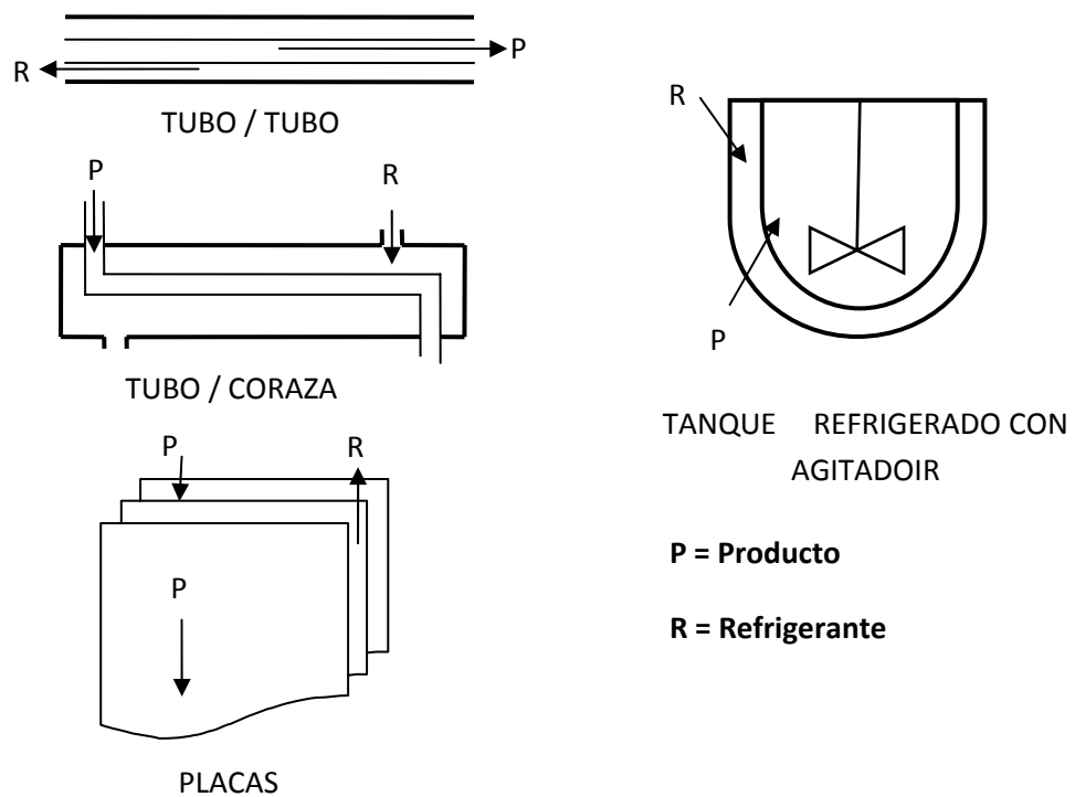
Figura 3.10 Esquema intercambiadores de calor.
