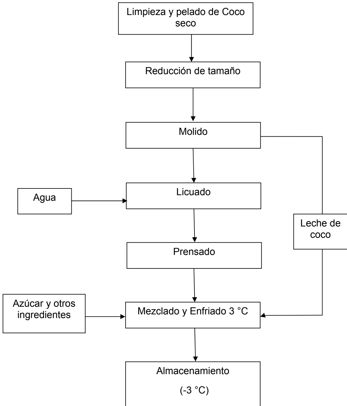
Figura 1.1 Diagrama de flujo de Proceso.
