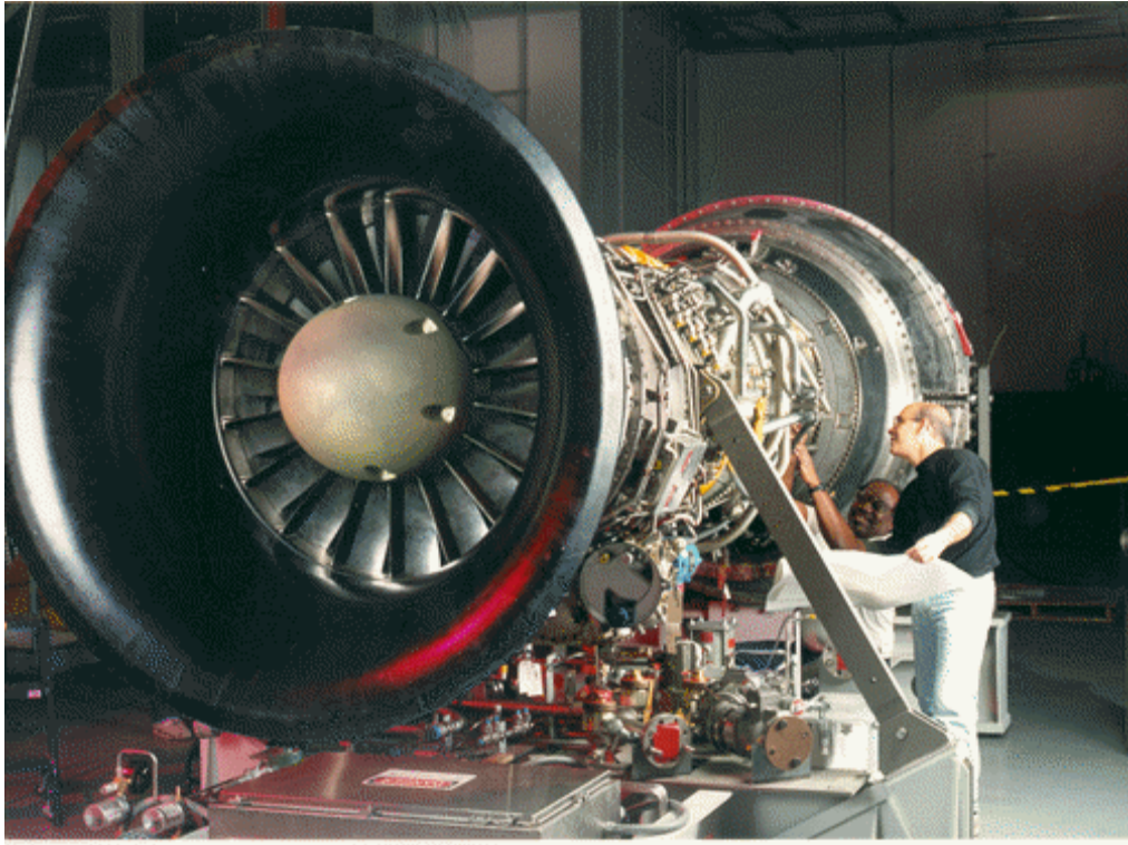
FIGURA 4.2. TURBINA A GAS AERODERIVADA
