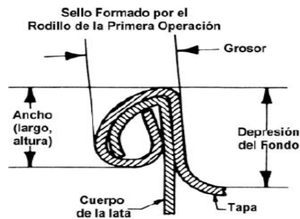
FIGURA 1.2: Primera operación de formado del doble cierre
