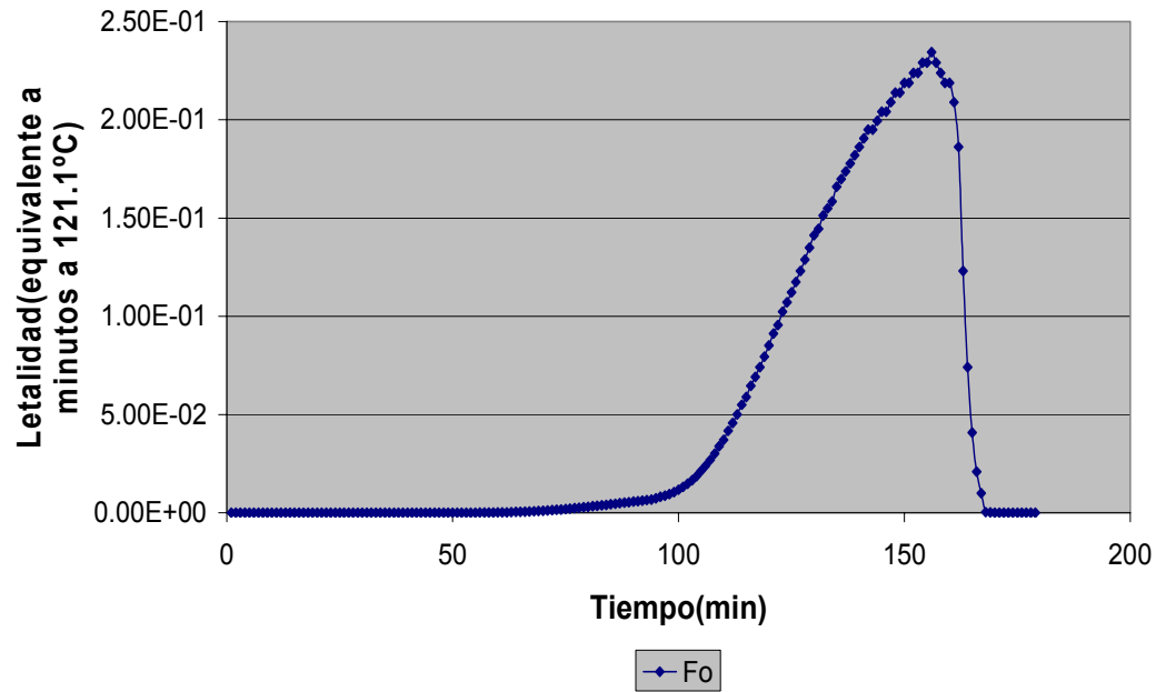
FIGURA 3.20: Letalidad vs. Tiempo, sensor M3P18271
