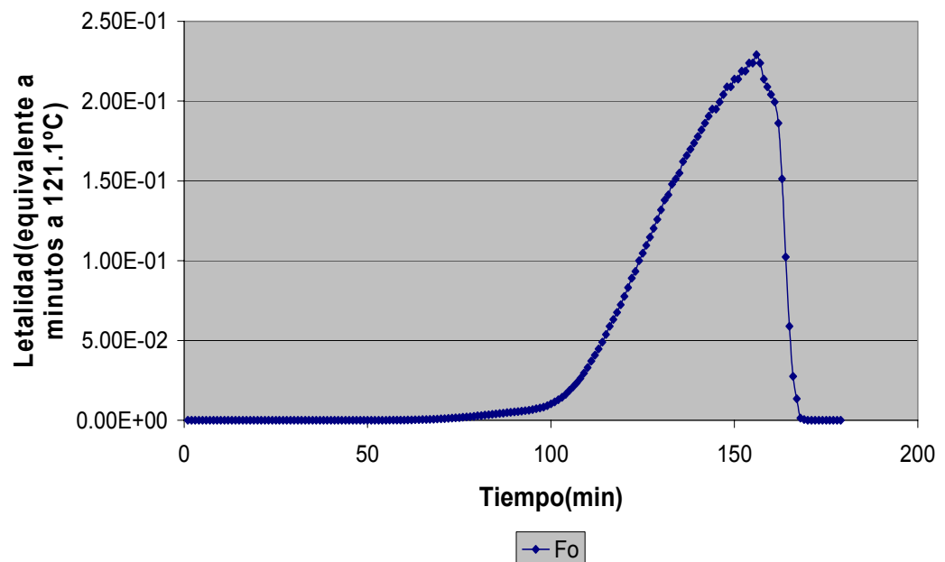
FIGURA 3.18: Letalidad vs. Tiempo, sensor M3P17494
