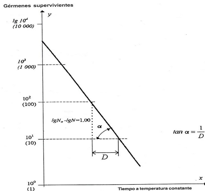
FIGURA 1.4: Curva logarítmica de supervivencia de los gérmenes
