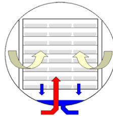
FIGURA 3.8: Entrada de vapor saturado y salida de condensado FUENTE: Sterilization retorts overview, 2004
