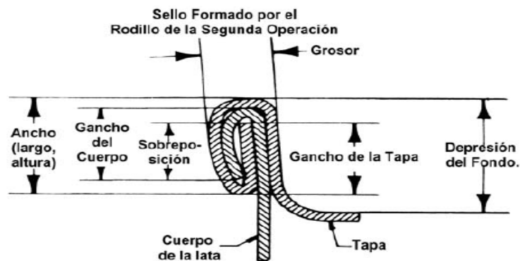
FIGURA 1.3: Segunda operación de formado del doble cierre
