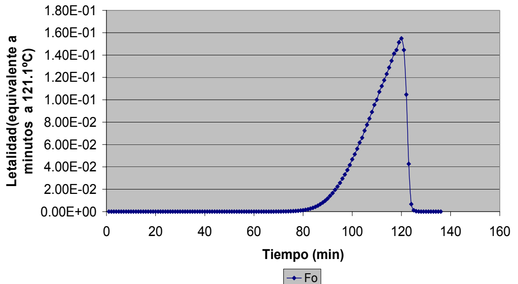
FIGURA 2.4: Letalidad vs tiempo (primer estudio de penetración de calor)
