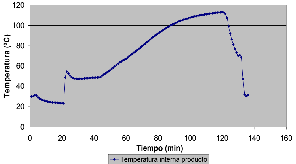
FIGURA2.3 Temperatura vs tiempo (primer estudio de penetración de calor)
