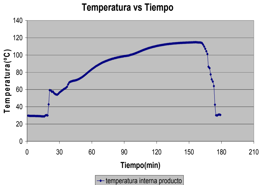
FIGURA 3.19: Temperatura vs. Tiempo, sensor M3P18271
