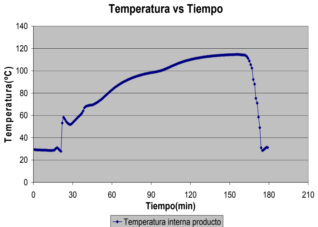
FIGURA 3.17: Temperatura vs. Tiempo, sensor M3P17494
