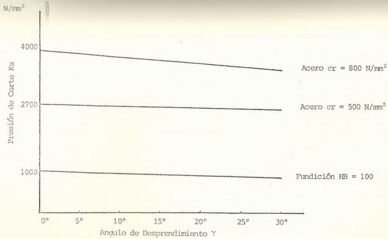
RELACIONES ENTRE LA PRESION Ks DE CORTE Y EL ANGULO DE DESPRENDIMIENTO
