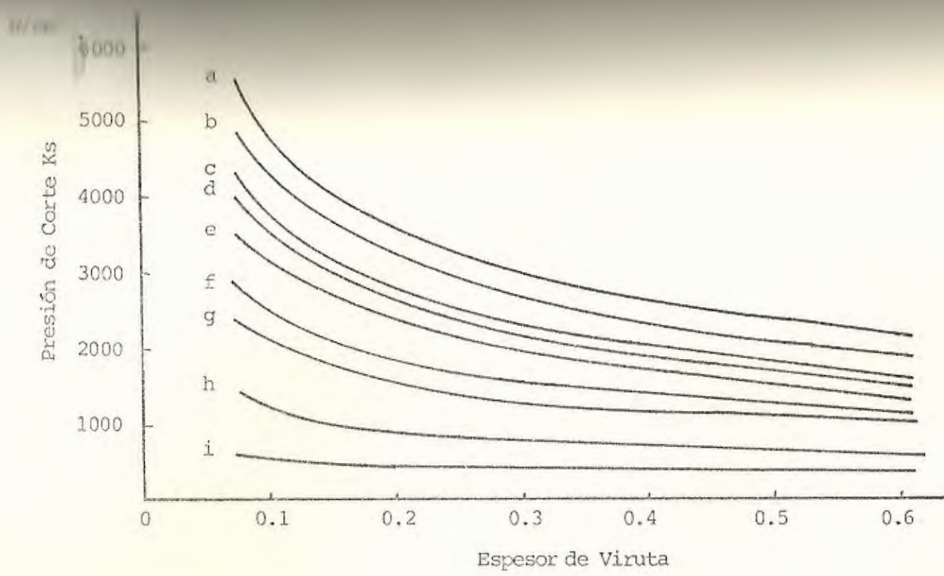
VARIACION DE LA PRESION DE CORTE, EN FUNCION DEL ESPESOR DE VIRUTA EN EL TORNEADO DE DIVERSOS MATERIALES
