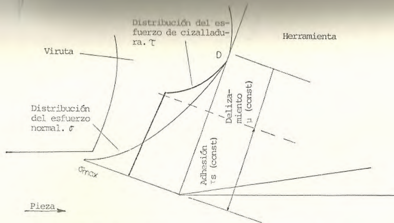
DISTRIBUCION DE ESFUERZOS EN LA PUNTA DE LA HERRAMIENTA DE CORTE
