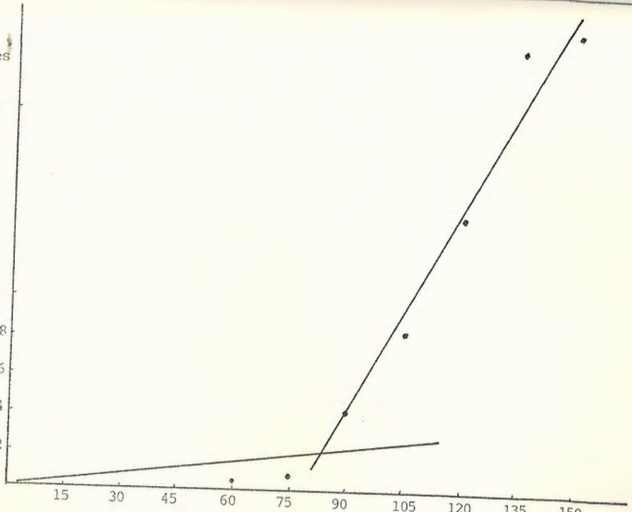
ENTALLE VS RUGOSIDAD UTILIZANDO LUBROREFRIGERANTE
