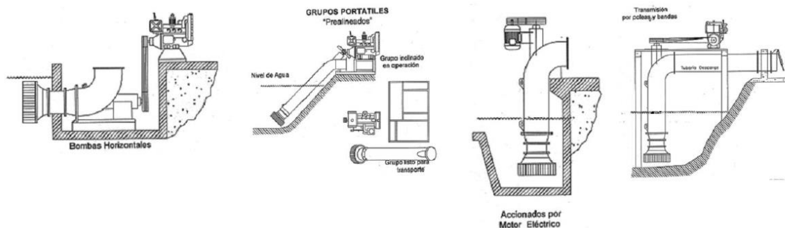
Ilustración 16 Diseño de Sistemas de Bombeo. Elaboración Pumpstek
