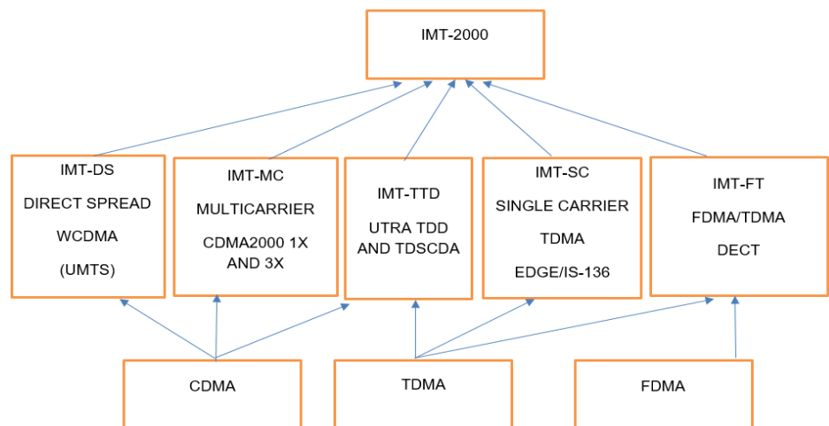
Figura 2.3.1: Estructura del Sistema IMT-2000 [9]
