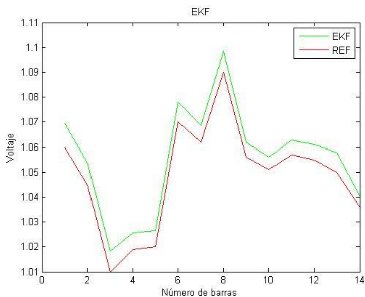
Figura 4.3: Voltaje vs Barra, Red 14 barras.
