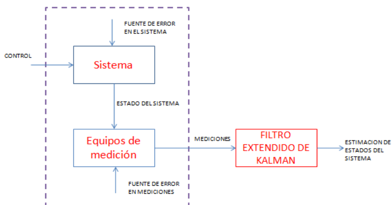
Figura 2.4 Aplicación típica del filtro de Kalman extendido.
