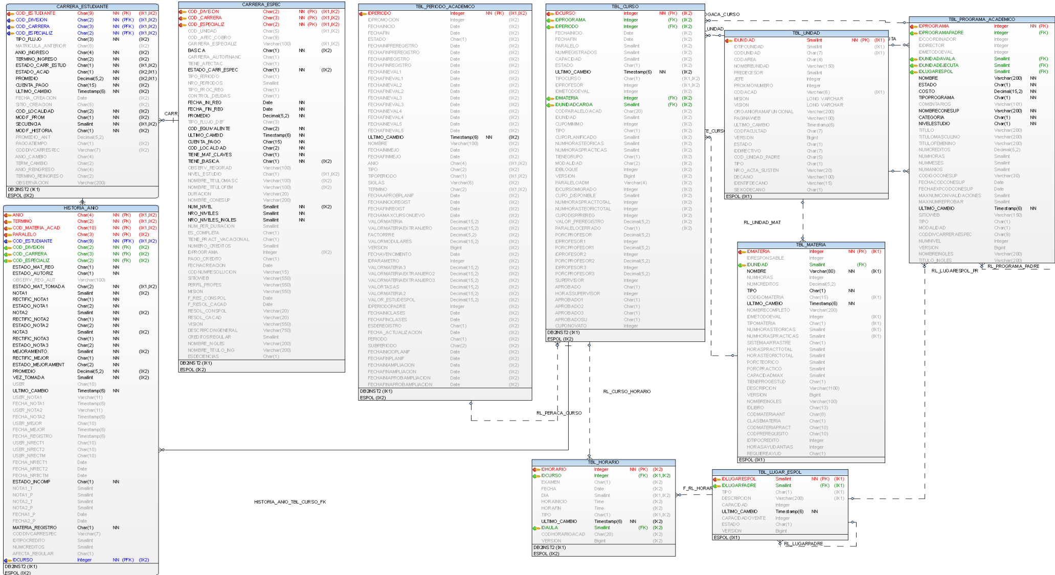
Figura 2.2 Modelo de datos académicos
